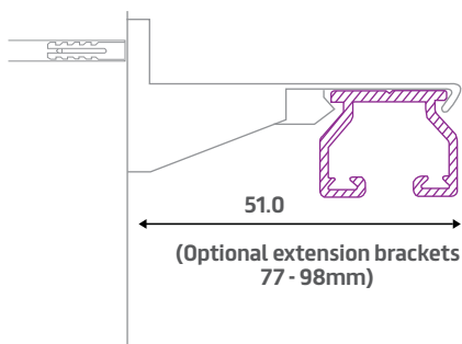
Face-fix
